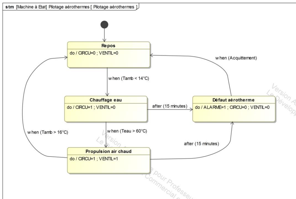
Diagramme d'états
