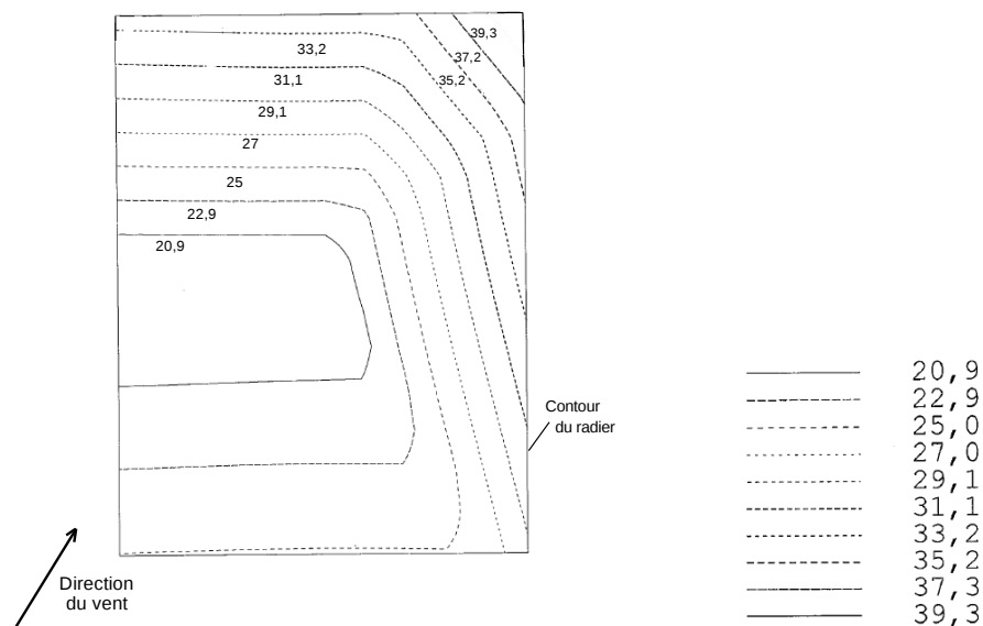
Simulation de la répartition des pressions exercées sur le sol en \text{kN} \cdot \text{m}^{-2}
