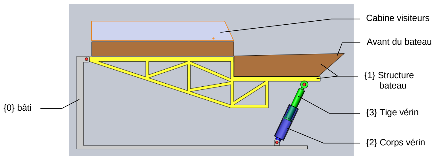
Position initiale
