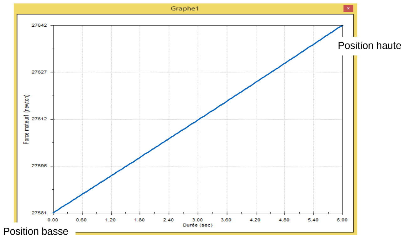
Simulation de l'effort fourni par le vérin
