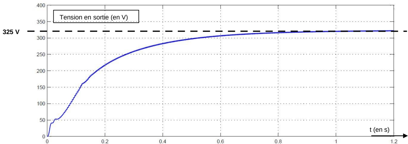
Tension en sortie du modulateur DC-DC
