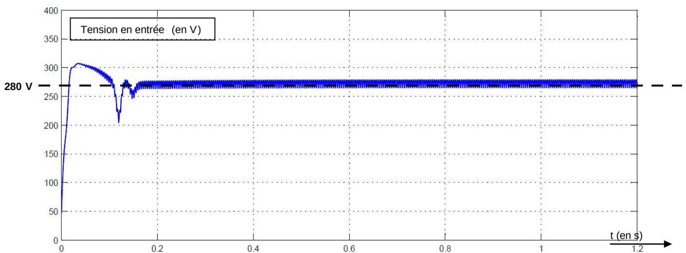
Tension en entrée du modulateur DC-DC
