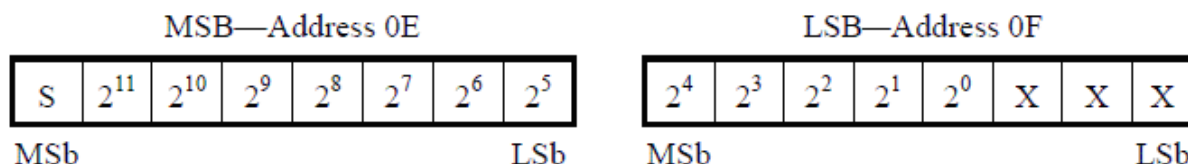
Format du registre « Current Register ».
