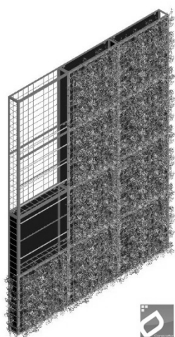
Structure d'un mur végétalisé
