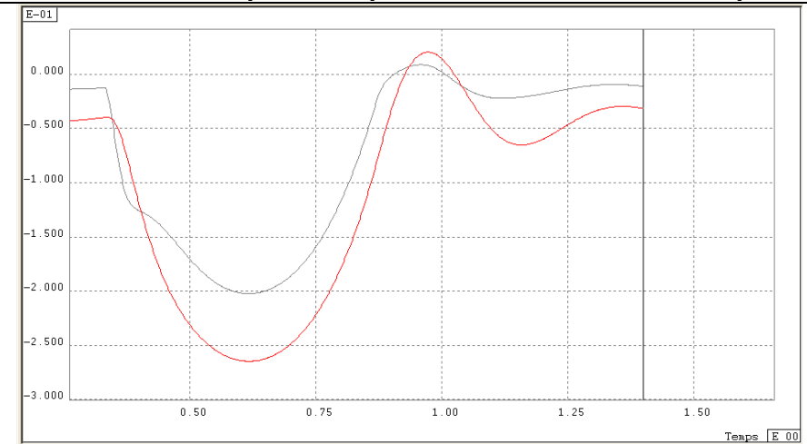
Cas 2 : Amortissement pour une pour une vitesse de 50 km/h (13.9 m/s)
